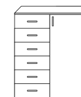
1 anta 6 cassetti 2 ripiani 101x120x35/45cm
